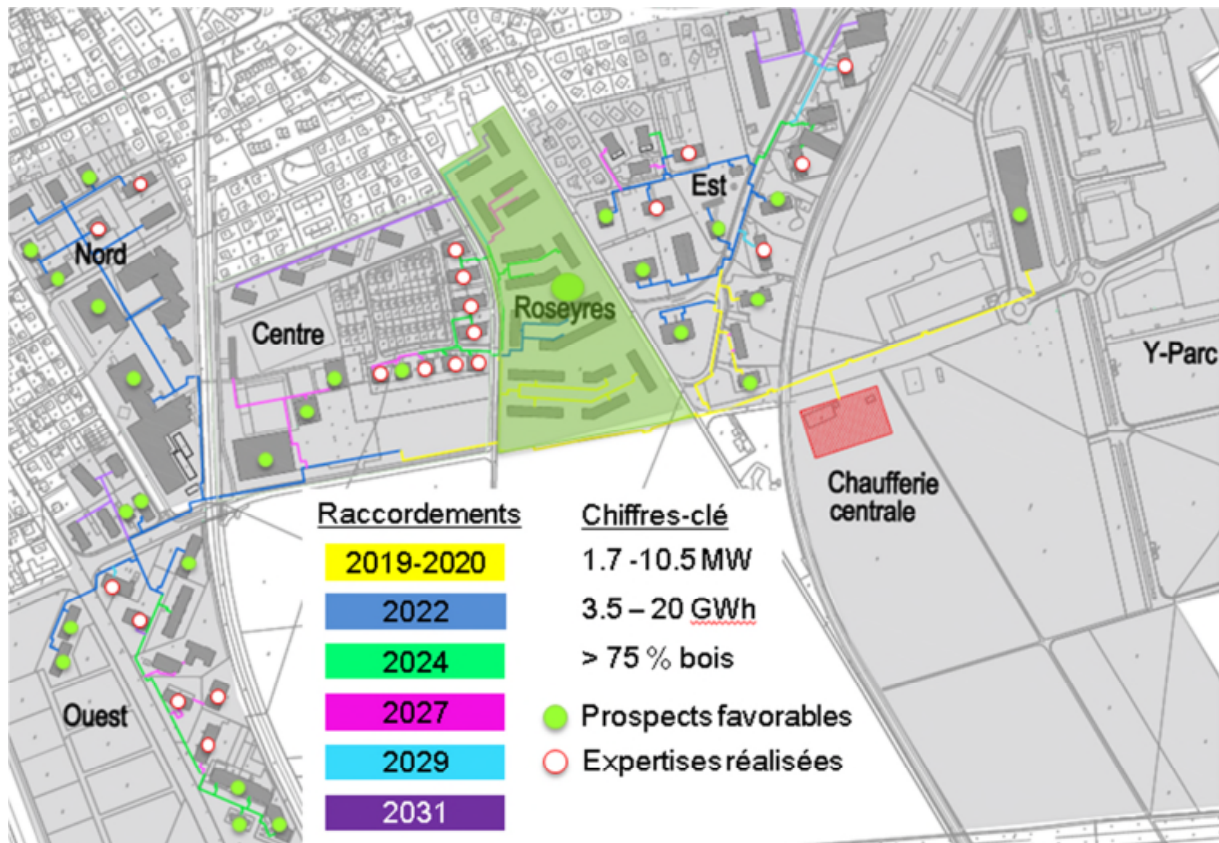
Figure 1 – Périmètre et planning de déploiement du CAD-SANTAL, y compris Y-PARC (2016).
