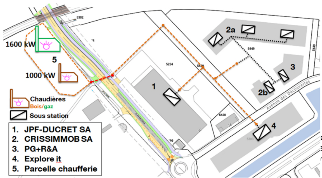
Figure 4 – Raccordement de l'îlot Y-PARC à la chaufferie bois-gaz via le réseau CAD-SANTAL, phase 2 : le PLAN « A » prévoit le financement de l'ensemble via CAD-SA, le PLAN « B » le financement de la chaufferie (5) par un contracteur, le réseau via la ligne n° 8044 du Plan des investissements.
