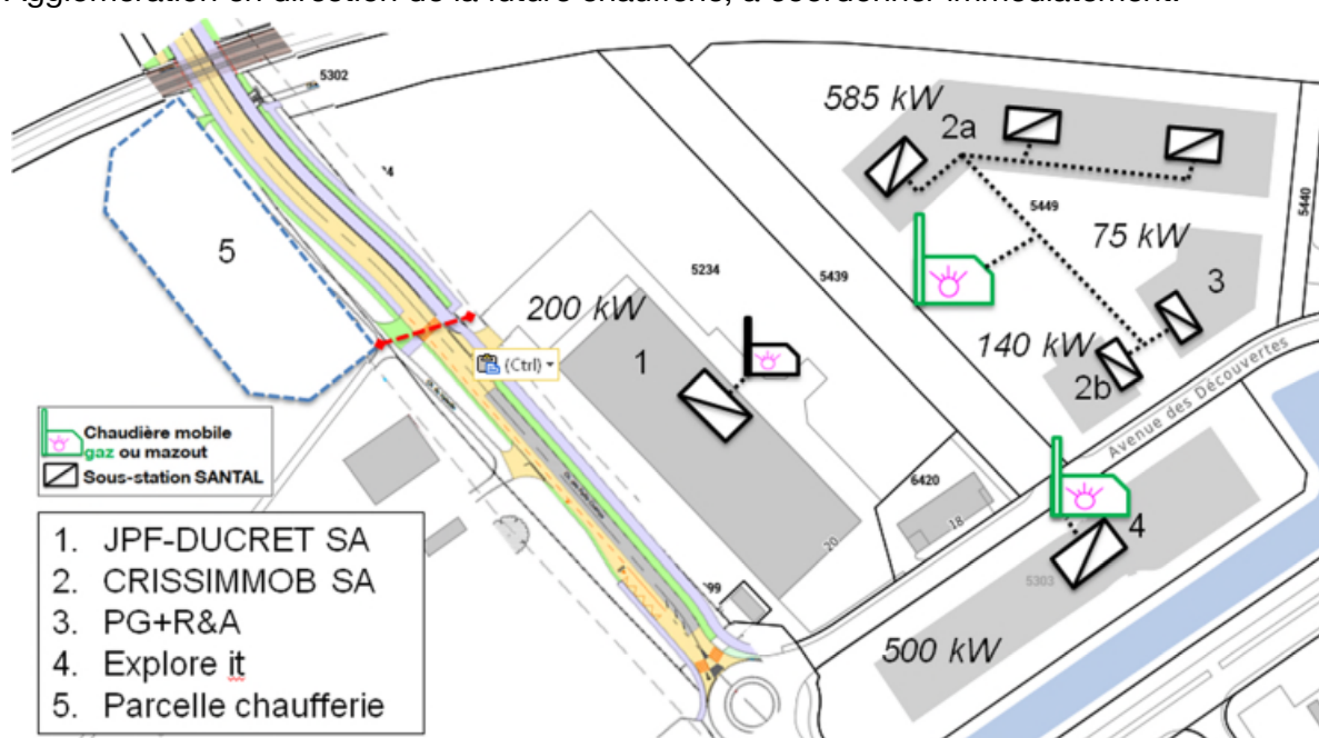
Figure 3 – îlot Y-Parc, phase 1 : tous les preneurs de chaleur sont alimentés jusqu'à la mise en service de CAD-SANTAL.
